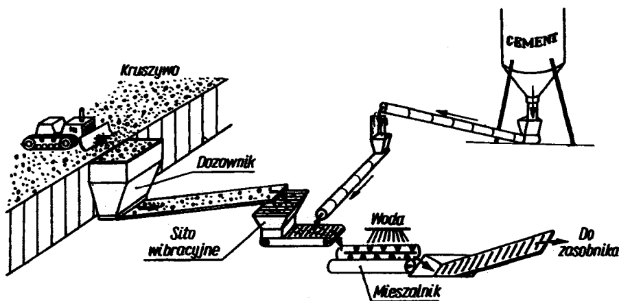
Rys. 7. Schemat technologiczny wytwarzania mieszanki kruszywa związanej cementem w mieszalnicach o działaniu ciągłym (wg: S. Rolla, M. Rolla i W. Żarnoch – Budowa dróg cz. 1. Wyd. Szkolne i Pedagogiczne, 1993)
