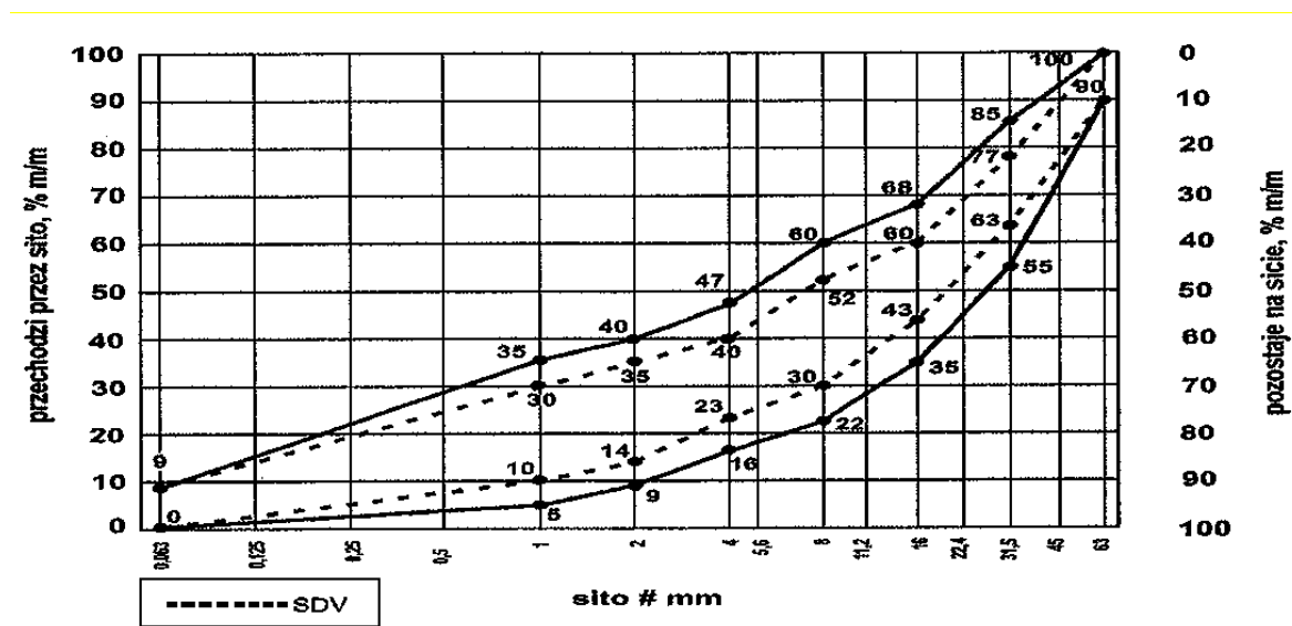
Rys. 1. Krzywe graniczne uziarnienia mieszanki kruszywa niezwiązanego 0/63 mm do warstw podbudowy zasadniczej
