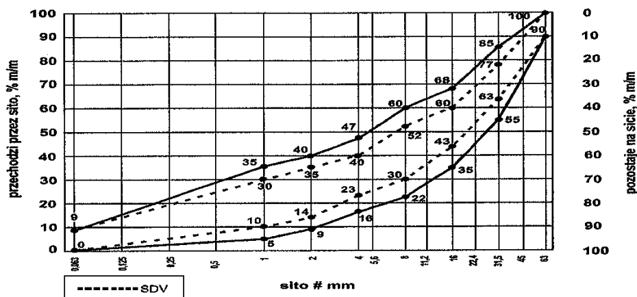
Rys. 1. Krzywe graniczne uziarnienia mieszanki kruszywa niezwiązanego 0/63 mm do warstwy podbudowy zasadniczej
